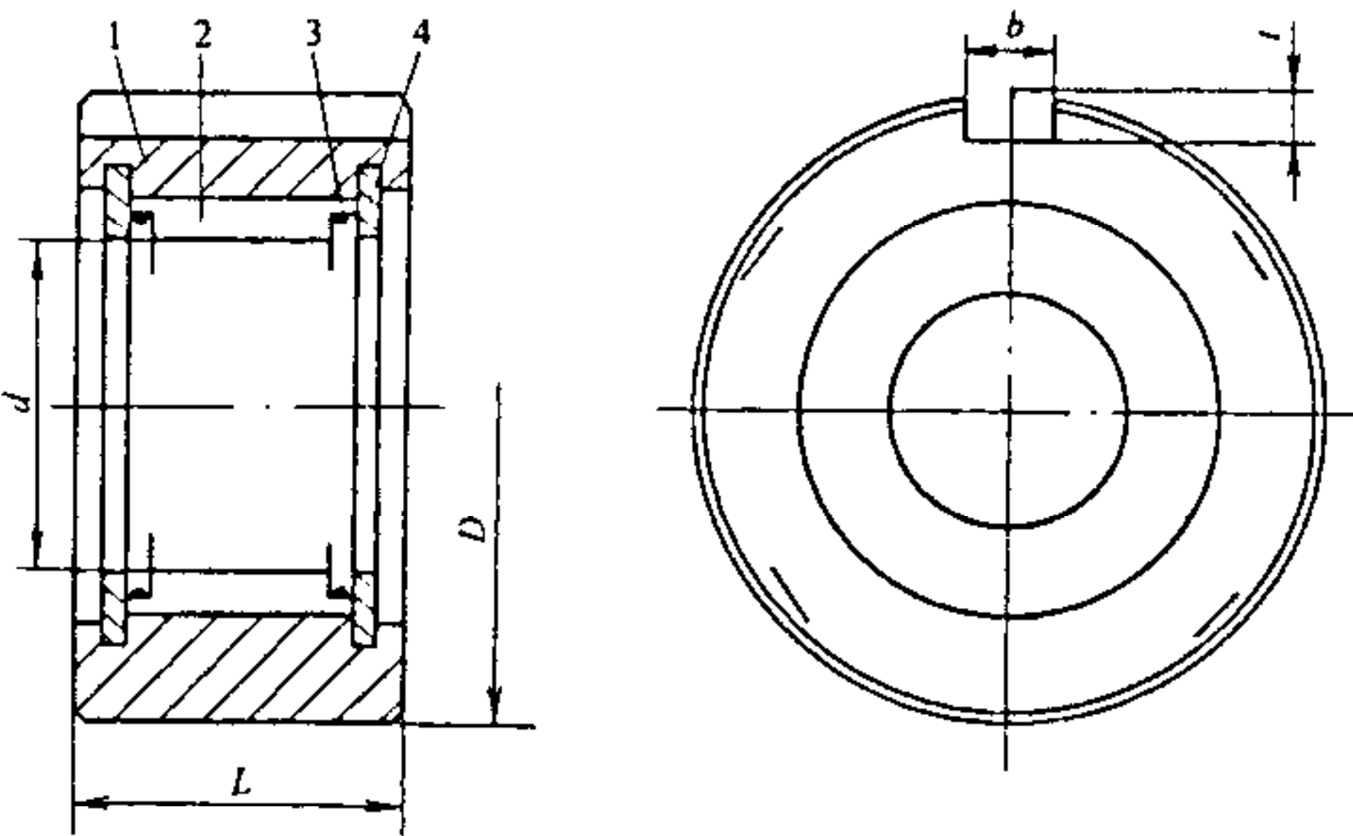
1——外环；2——楔块；3——弹簧；4——端盖。
