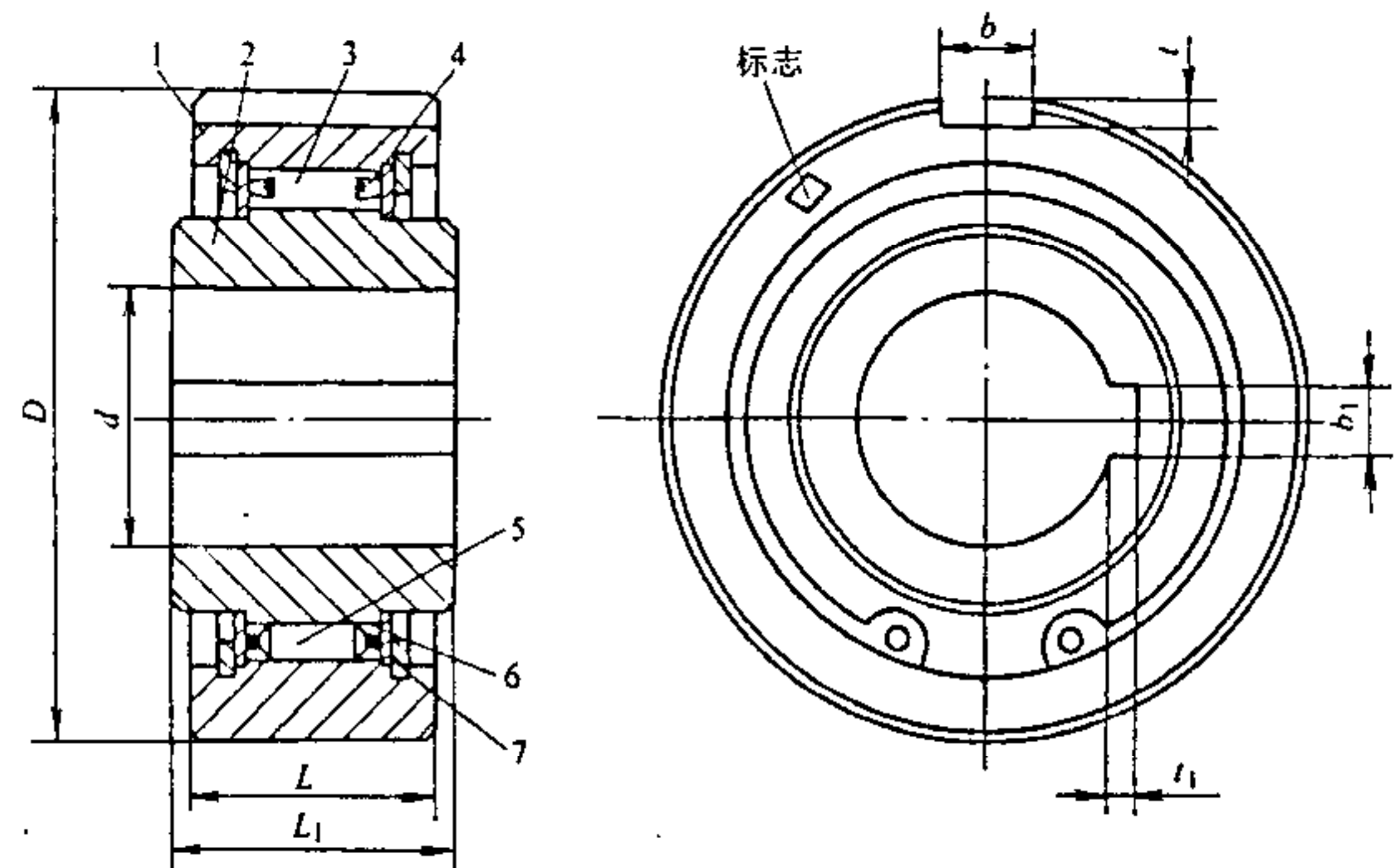
1——外环；2——内环；3——楔块；4——弹簧；5——滚柱；6——端盖；7——挡圈。
