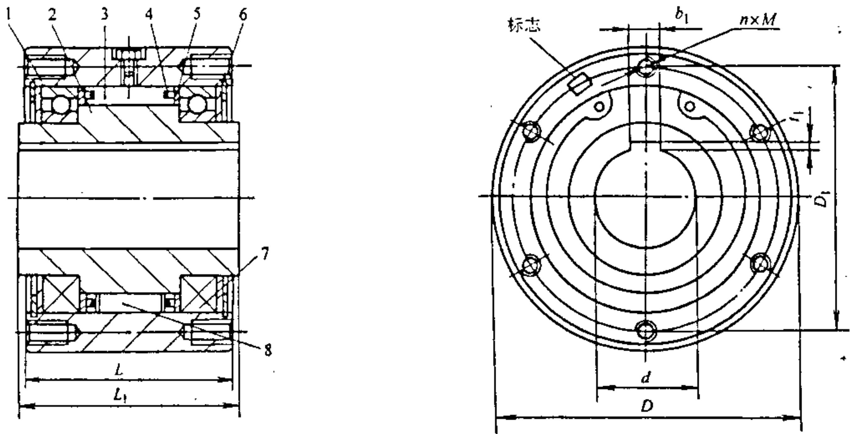
1——外环；2——内环；3——楔块；4——弹簧；5——垫圈；6——端盖；7——轴承；8——滚柱。
